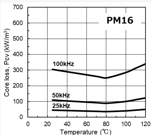
【コアロスの温度依存性(Bm=200mT)】
