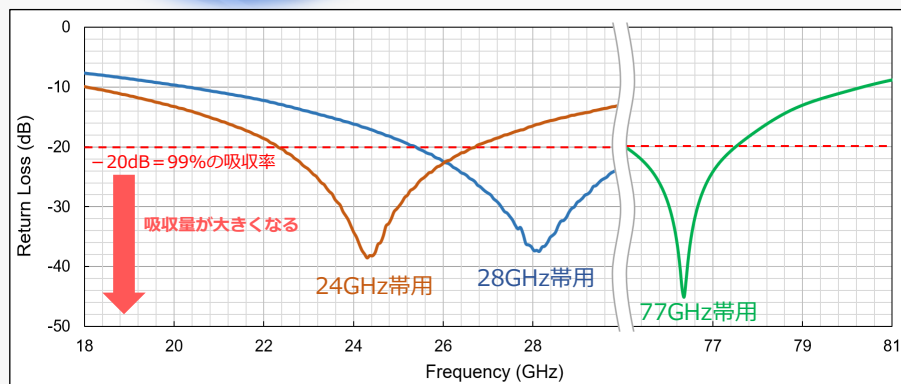
【ミリ波電磁波吸収シートの性能】
